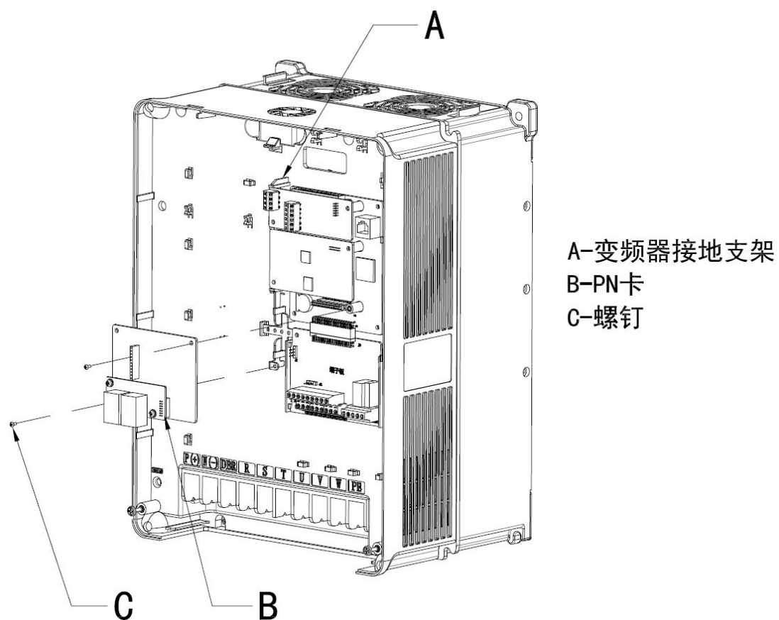
图 1 PN 卡的安装与接地
