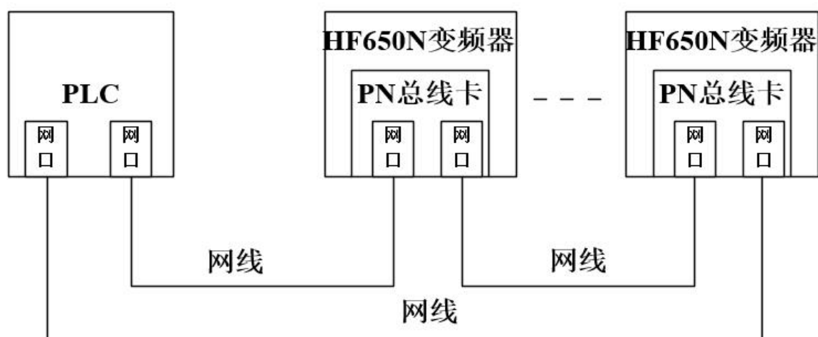
图 2 标准 PROFINET 环网电缆接线图
