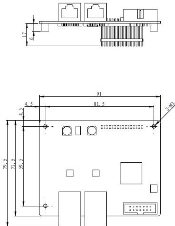
图 5 PROFINET 模块尺寸 (单位 mm)
